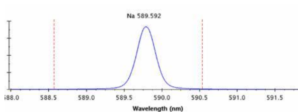
4-rasm. Plazma optik emissiya spektroskop tahlili
